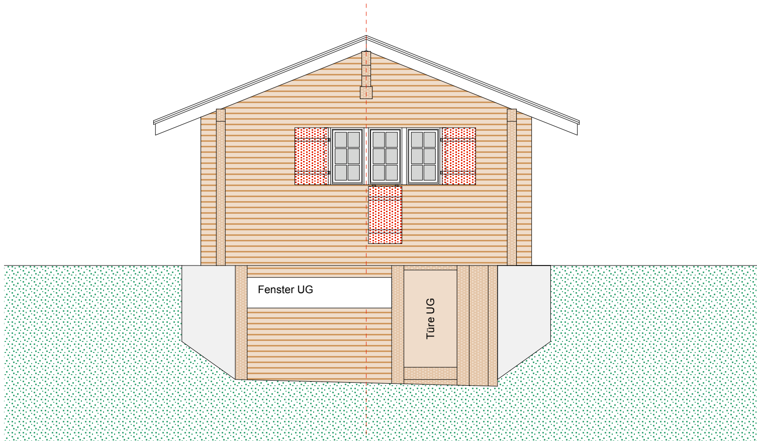
Südfassade
